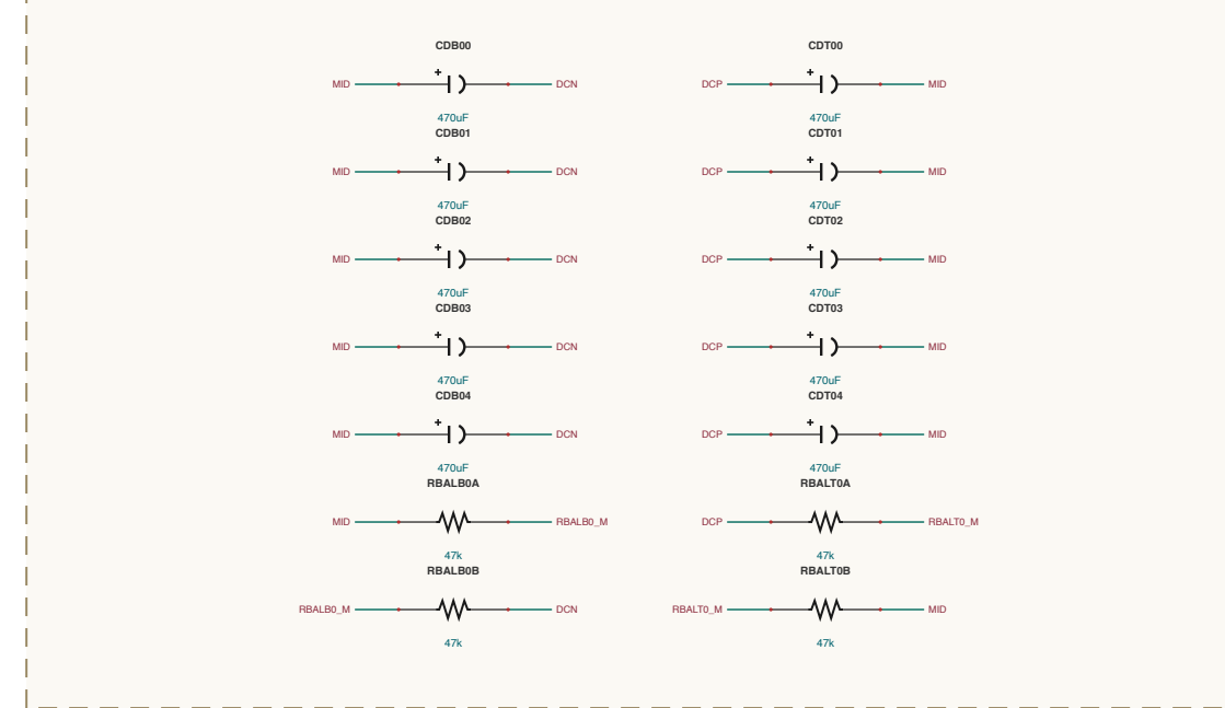
DC-LINK / LINK-BANK-0
