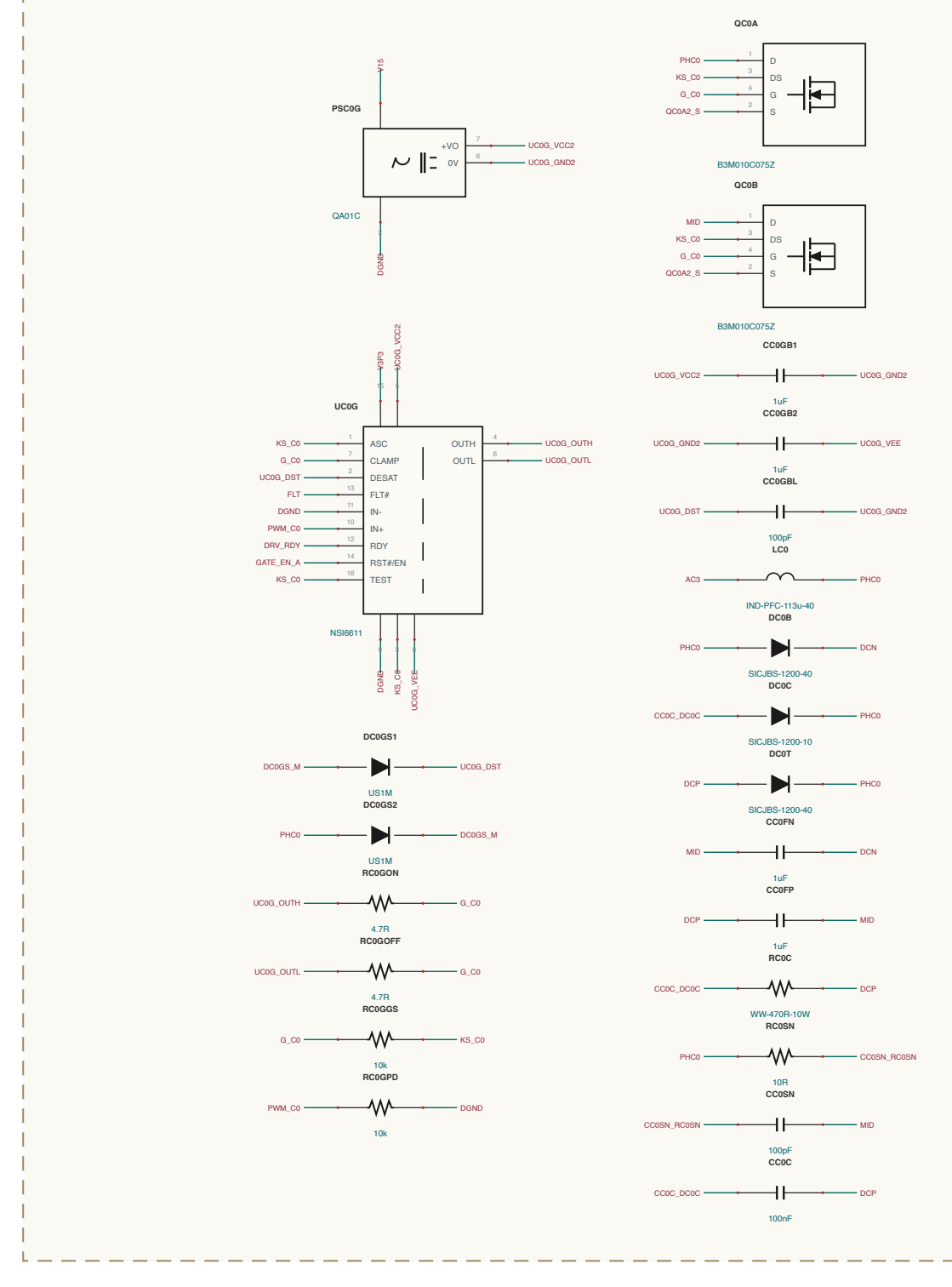
VIENNA-PFC / PHASE-C0
